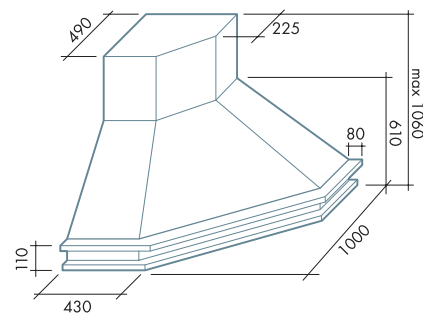
angolo/wall corner
